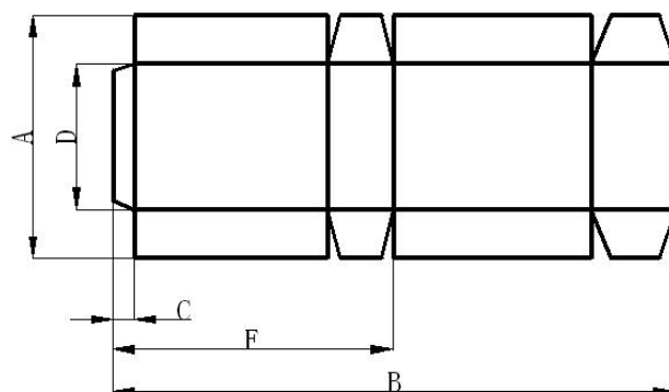
平口纸箱示意图
